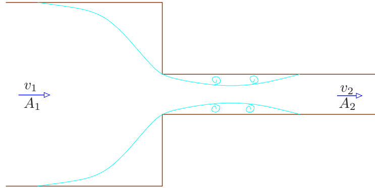
Figura 21.7: Contracción brusca.
