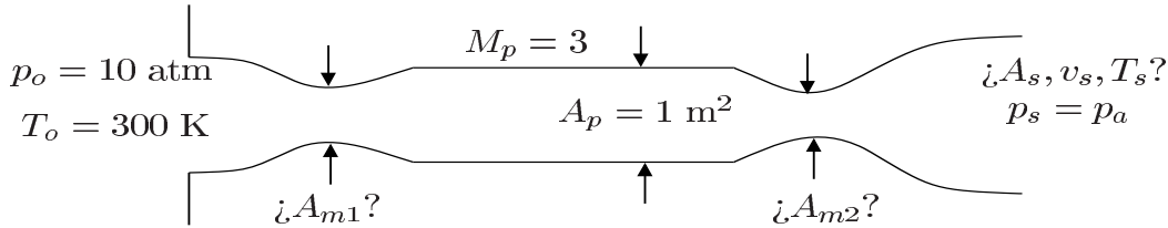
Figura 18.23: Túnel aerodinámico
