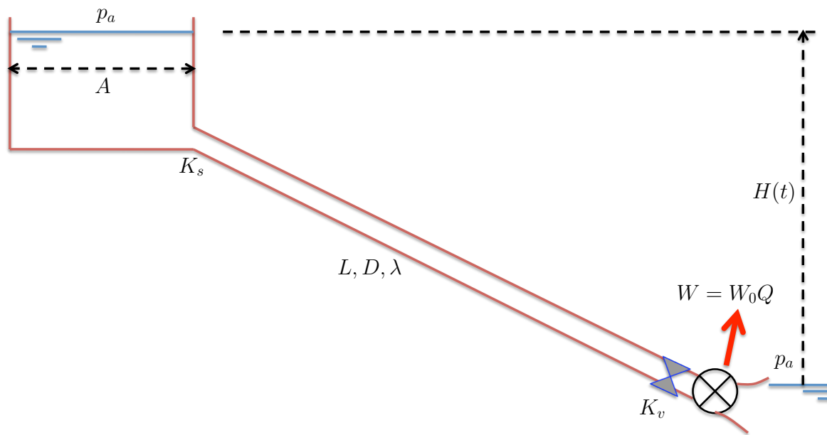
Figura 21.29: Miniturbina.
